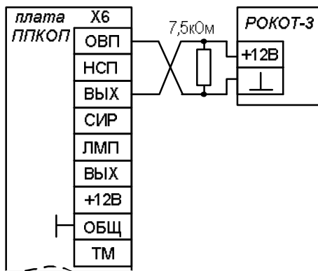
Рис.2 Схема подключения к приборам «Гранит-16/24», «Пирит», «Карат»
